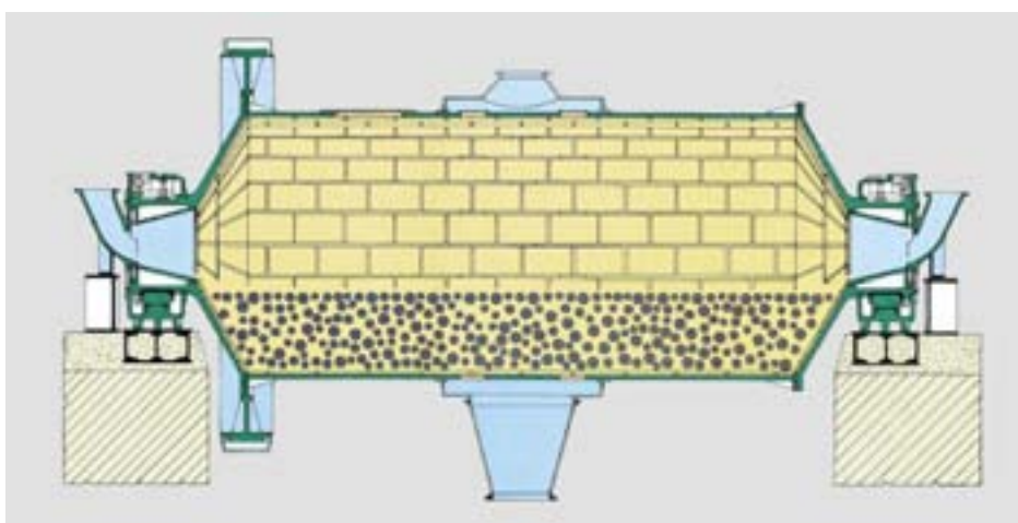
Bi-broyeur à boulets avec décharge central
