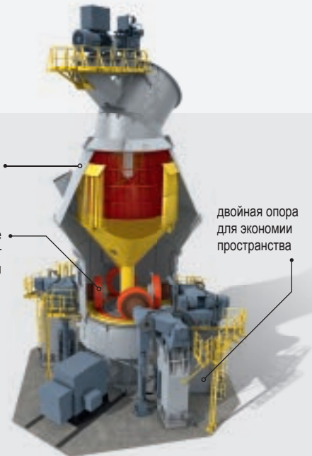
Мельница MVR
